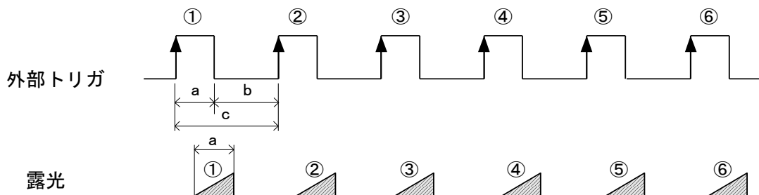
図 4-5-3-1 外部トリガ (TriggerWidth) 露光モード
