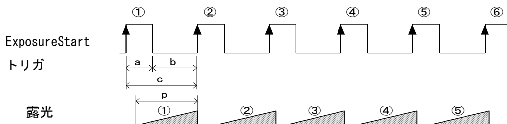
図 4-5-2-1 外部トリガ (Timed) 露光モード
