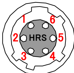
図 3-3-1 カメラ側電源コネクタ（ヒロセ：HR10G-7R-6PB）
