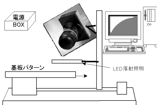
図 1-2-2 プリント基板の外観検査装置
