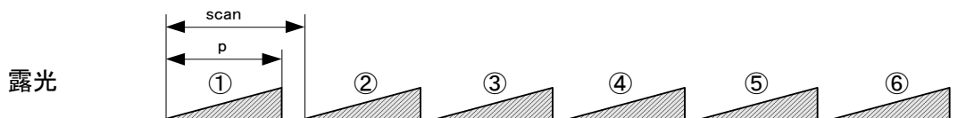
図 4-5-1-1 フリーラン露光モード
