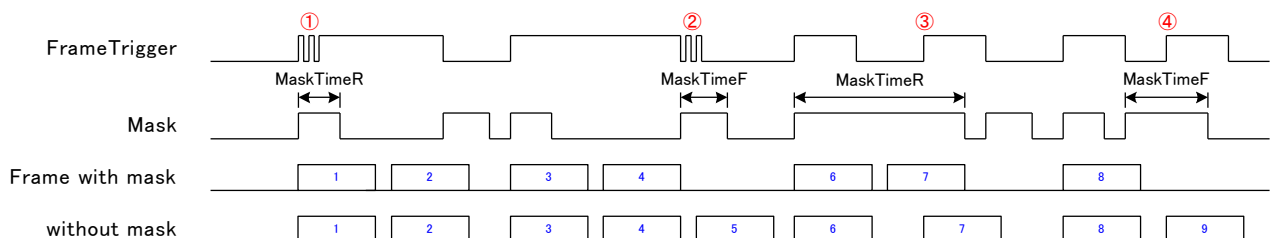
図 4-2-6-1 外部フレームトリガ入力とマスクの効果
